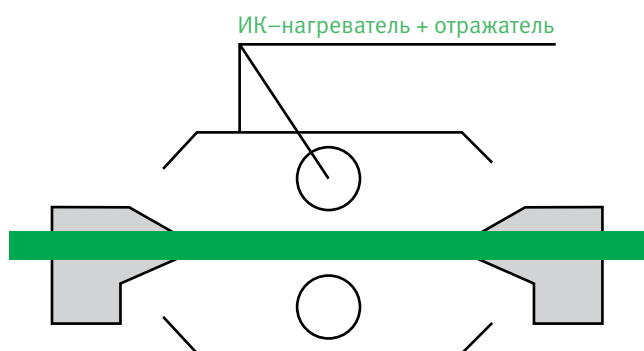
Рисунок 5. Горячий линейный изгиб. Стекло Novattro® должно местно нагреваться с помощью ИК-излучателей или провода сопротивления.
