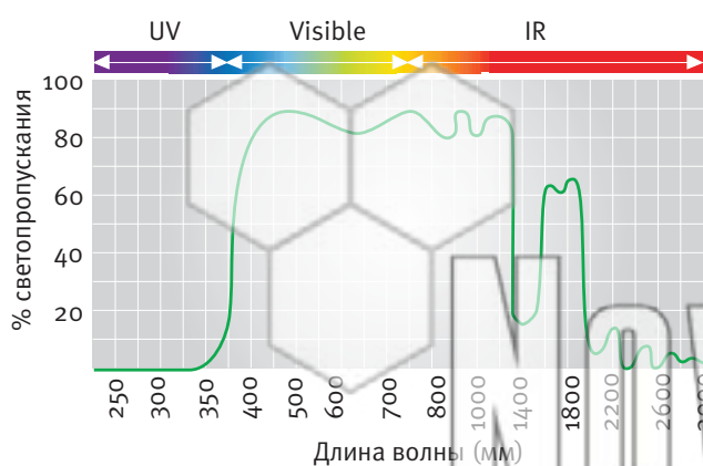
График 1. Процент светопропускаемости полимерного стекла Novattro® (толщиной 3 мм) относительно длины волны
